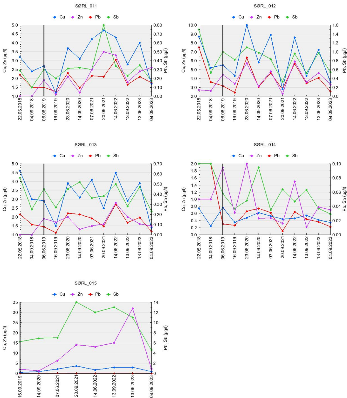
Figur v1b. Konsentrasjoner av bly (Pb), kobber (Cu), sink (Zn) og antimon (Sb) i punkter på Sørليا SØF. Fra og med 2019 ble det analysert på filtrerte prøver, og overgangen fra ufiltrerte til filtrerte prøver er angitt med sort vertikal linje.
