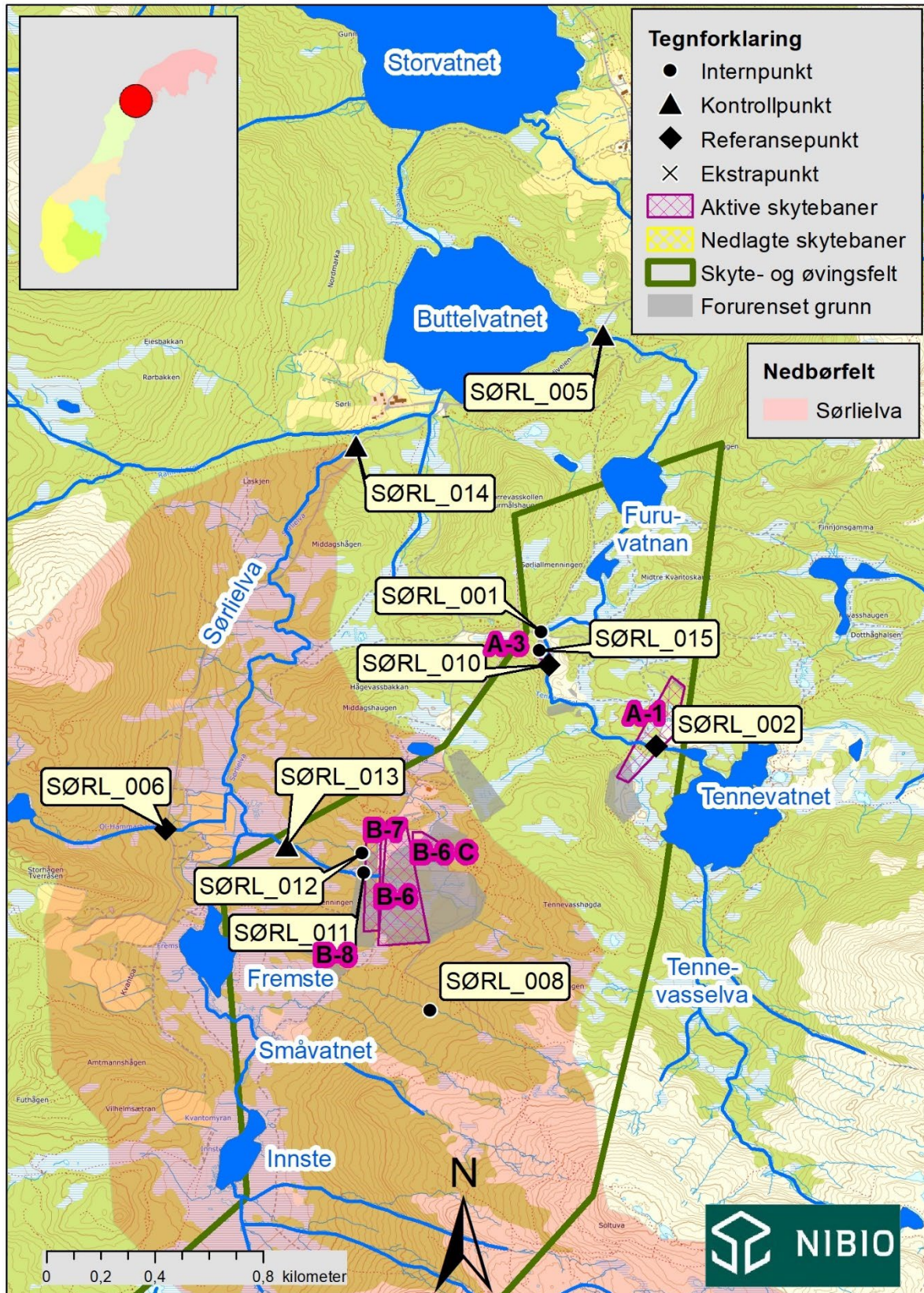
Figur 1. Prøvepunkter med delnedbørfelt på Sørlielva SØF i 2023.
