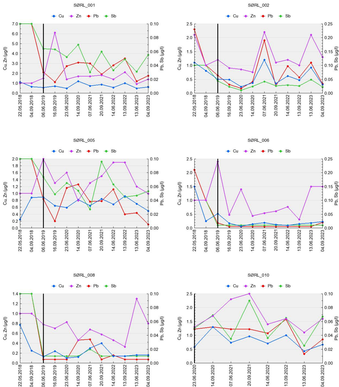
Figur v1a. Konsentrasjoner av bly (Pb), kobber (Cu), sink (Zn) og antimon (Sb) i punkter på Sørlia SØF. Fra og med 2019 ble det analysert på filtrerte prøver, og overgangen fra ufiltrerte til filtrerte prøver er angitt med sort vertikal linje.
